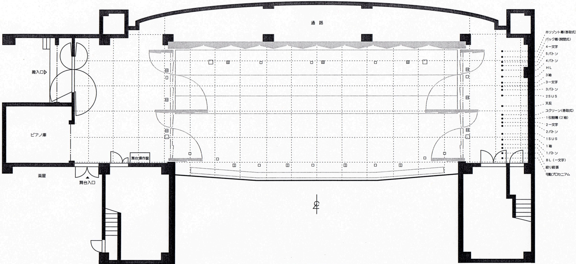
舞台平面図 1/100
